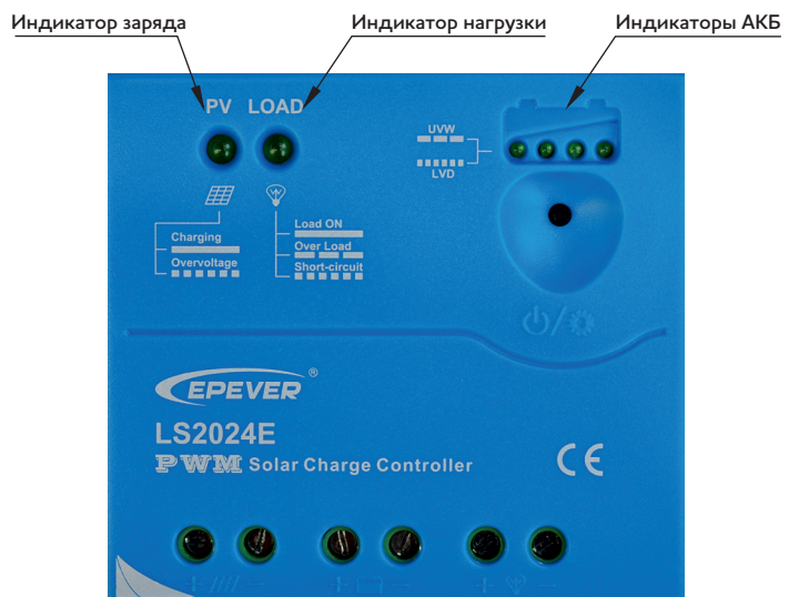
Рисунок 3. Светодиодные индикаторы.
